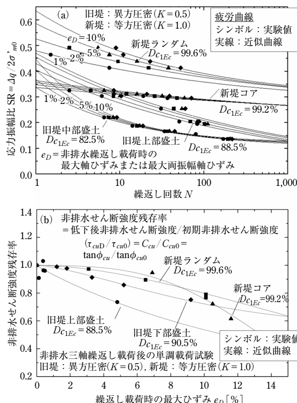
図-8 新旧堤の堤体材料の疲労曲線とせん断強度低下特性 12)
