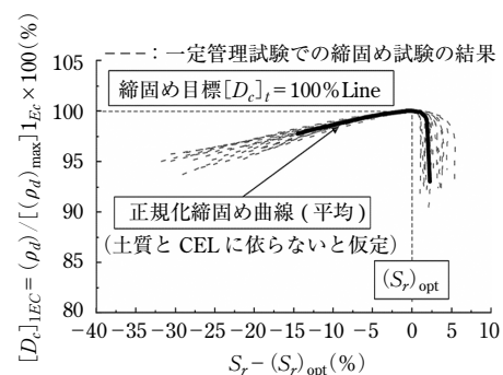
図-4 正規化締固め曲線(新堤体の遮水ゾーンでの例) 3)
