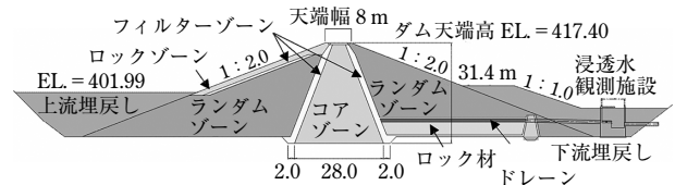
図-2 新本堤(中心遮水型アースフィルダム)
