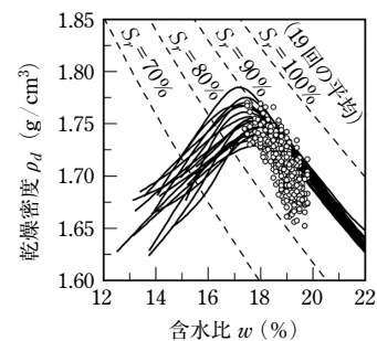
図-3 新本堤の遮水ゾーンでの19回の定期管理による1Ecでの締固め曲線と現場締固め状態の全データ 3)
