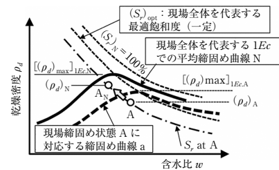
図-6 実測締固め状態から等価な締固め状態への変換方法 3)
