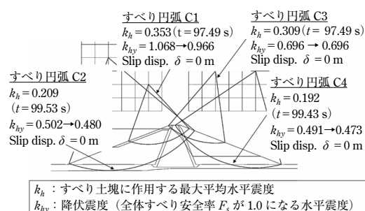
図-9 新本堤のNewmark-D法と非線形FEMによる地震時残留変形解析
