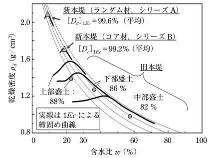
図-1 旧本堤と新本堤の締固め特性と締固め度 [D_c]_{1Ec}
