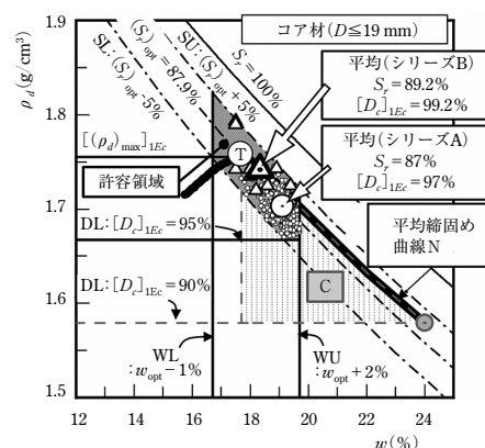
図-5 新本堤の遮水ゾーンの締固め曲線のばらつきを除去した全定期管理試験（剪頭粒度試験試料）のまとめ
