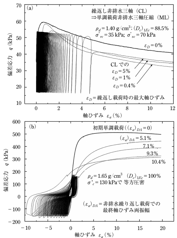
図-7 三軸実験による飽和盛土材の非排水せん断強度の非排水繰返し载荷による低下の例 (a: 旧本堤上部盛土試料(緩詰め), b: 新本堤コア試料(密詰め)) 13)
