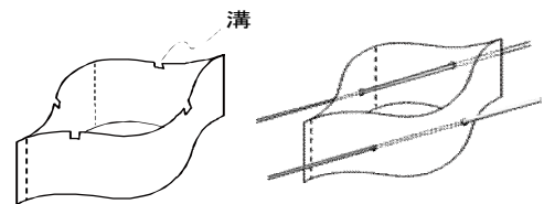
図4.1 セル部に鉄筋類を通す方法の1例 <参考文献>1) 松丸貴樹・小島謙一ら：降雨の影響を考慮した盛土の棒状補強材を用いた耐震補強対策工の検討，第43回地盤工学発表会，pp1147～1148，2008年 2) 松丸貴樹・小島謙一・館山勝ら：模型実験による背面地山の浸透水を受けた盛土の耐震対策工の評価，第43回地盤工学発表会，pp1149～1150，2008年
