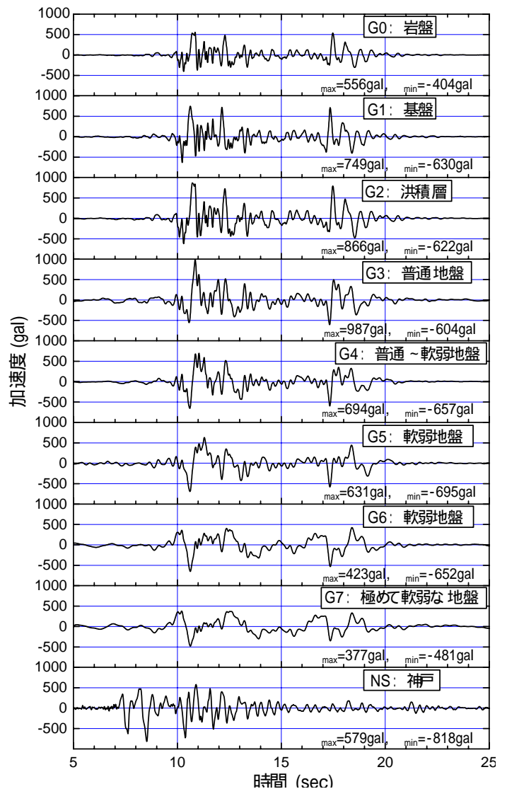
図-1 新耐震標準の適合波形 (G0~G7)
