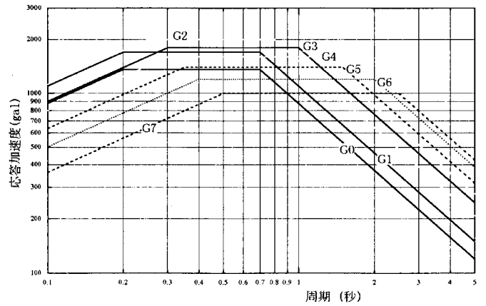
図-2 各地盤種別の地表面での弾性加速度応答スペクトル (スペクトル)
