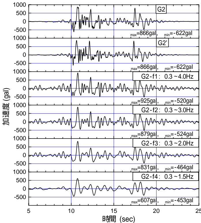
図-4 修正した適合波形 (G2)
