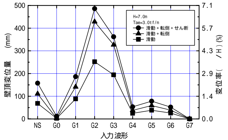
図-3 地盤区分と変位量の関係
